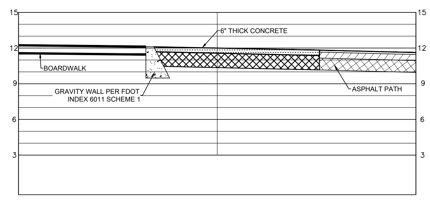
SECTION D-D SCALE: 1" = 5'
